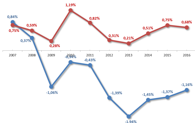
Tasso crescita imprese totali e artigiane periodo 2007-2016
