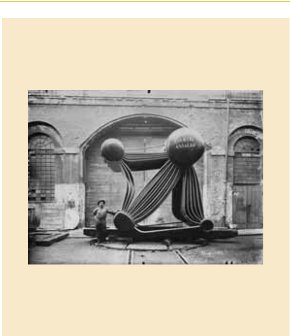
Caldaia nello stabilimento Meccanico Ansaldo di Sampierdarena (1913)
